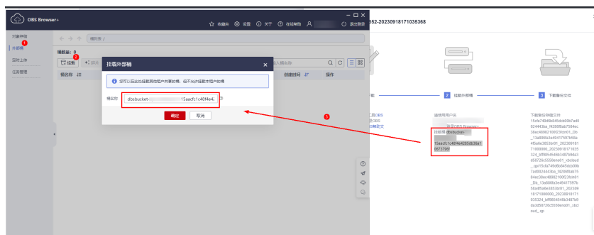
图 7-7 挂载外部桶
