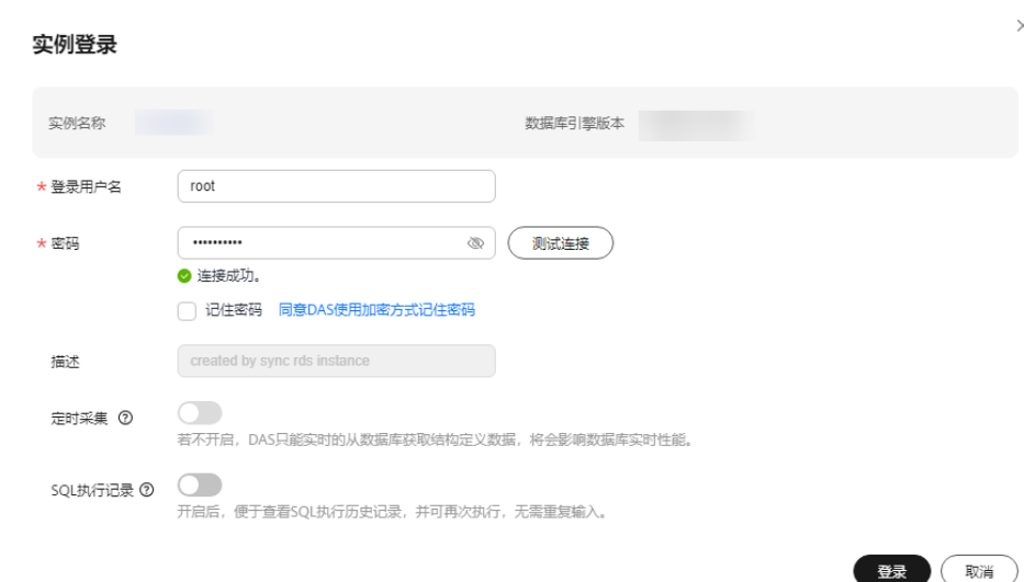
图 3-3 登录界面
