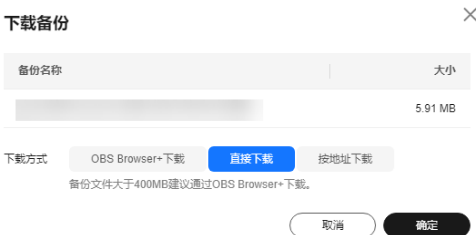
图 7-9 直接下载
