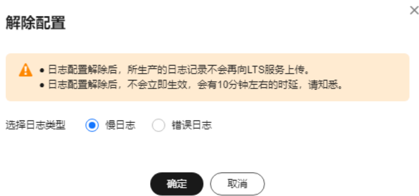
图 13-3 解除配置
