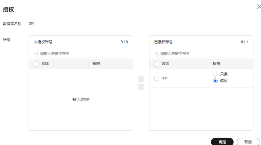
图 4-2 数据库授权
